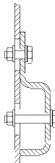
Fig. 2. Infästning av plankan med dubbla bultar
