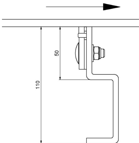
Fig. 1. Avskraparplankan +250° monterad under returparten
